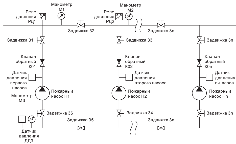
Рис. 8 Общая принципиальная схема установки Hydro-FS-A
